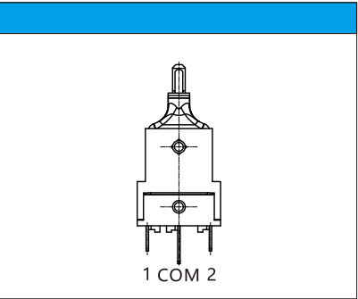
■外形尺寸
