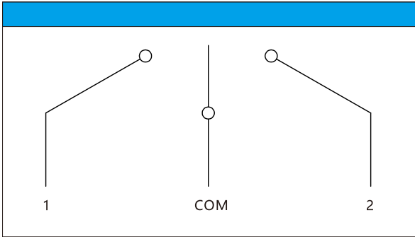
■接触形式图
