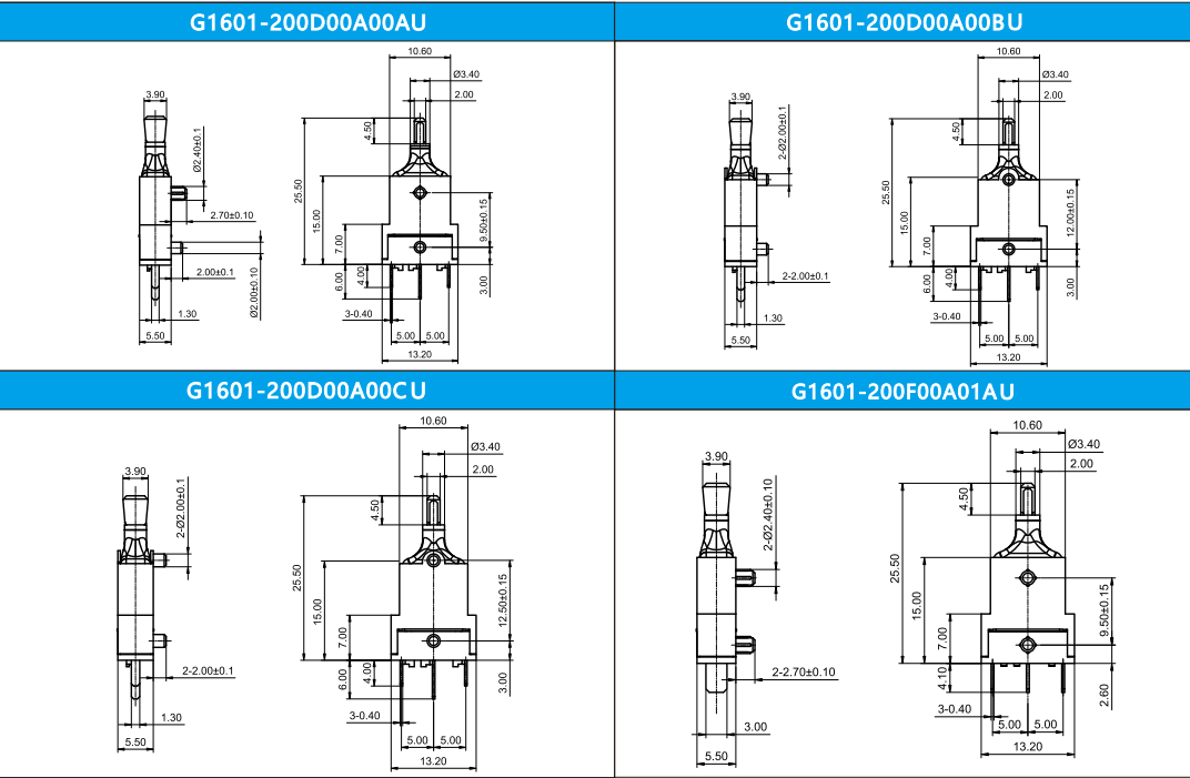
■外形尺寸
