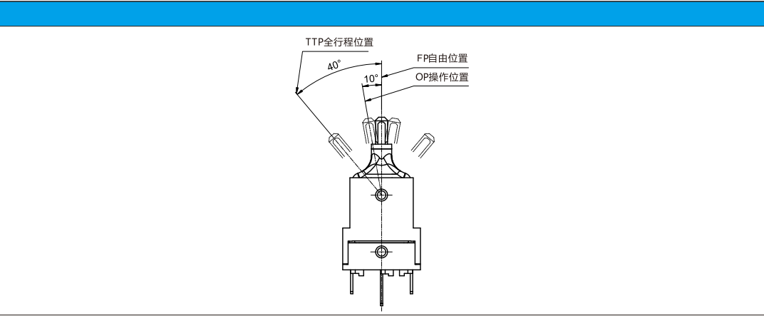
■操作特性图
